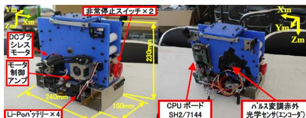
図1 開発したメーセイスペースエレベーターⅠの概要
