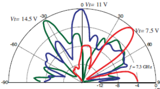
図4 放射パターンの測定結果
