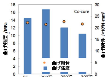
図3 曲げ特性
