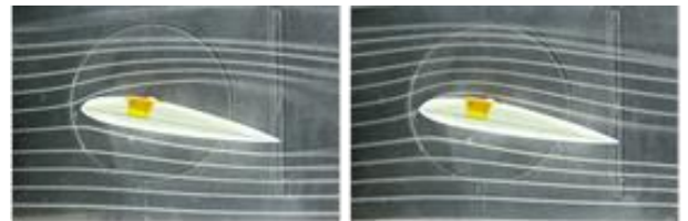
図3 プラズマ・オフ 翼失速 プラズマ・オン 飛行回復
