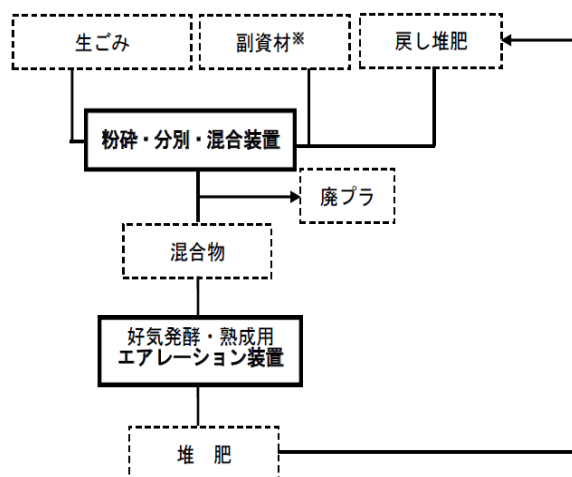
図1 堆肥化システムの処理フロー
