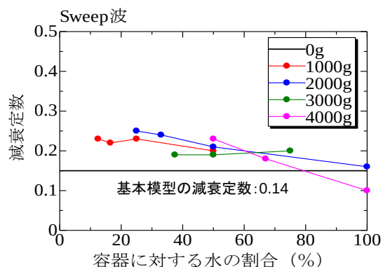
図2 スイープ実験における減衰定数
