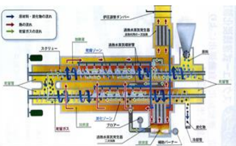
図1. 連続式炭化炉(横型スクューキルン)
