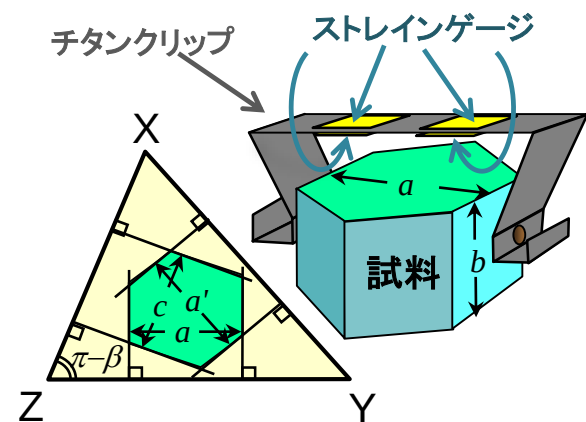
図1 クリップ型ストレインゲージ熱膨張計による単斜晶系試料の測定（ a 軸方向の測定例）
