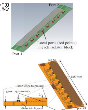
図2 電磁界モデル (上) と放射ビーム走査漏洩波アンテナ (下)
