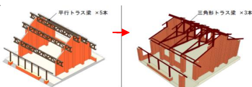
図4 トラス梁の変更
