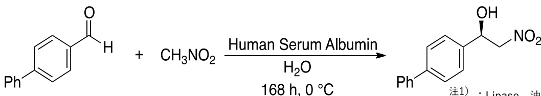
図2 ニトロアルドール反応（ヘンリー反応） 単離収率70%、エナンチオマー過剰率79%
