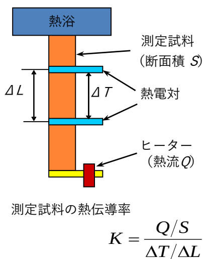
(a) 定常熱流法
