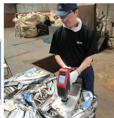
可搬型蛍光X線分析装置による現場分析（塗装剥離後に測定）
