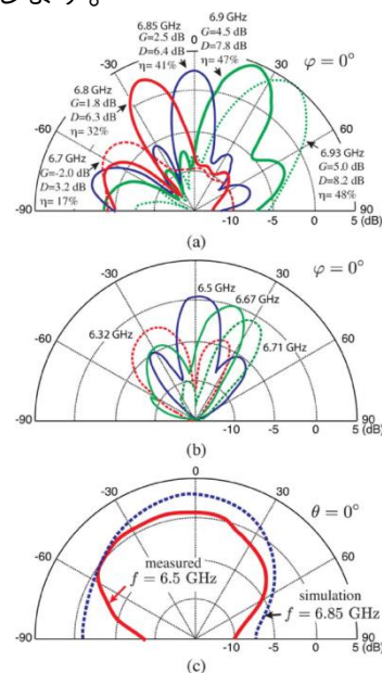
図4 漏洩波アンテナ放射パターン
